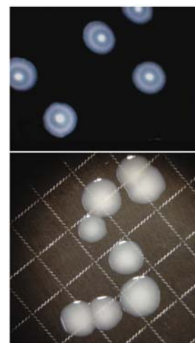
Bild 3. Kolonien von Legionella pneumophila Serogruppe 1 direkt auf Agar (oben) und Legionella pneumophila Serogruppen 2 bis 15 auf schwarzem Membranfilter (unten); stereomikroskopische Aufnahmen (die Größe einer Kolonie beträgt etwa 5 mm)
